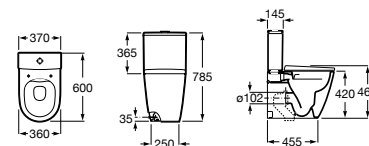
Inodoro de tanque bajo compacto adosado a pared 600 mm de longitud
