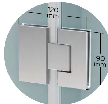
Detalle de bisagra vidrio-vidrio Aluminio-Zamak
