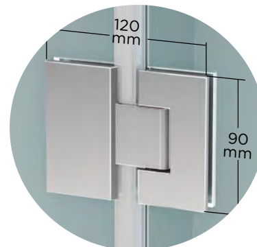
Detalle de bisagra vidrio-vidrio Acero Inoxidable
