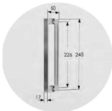
Tirador Aluminio-Zamak
