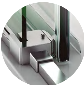
Detalle guía inferior
