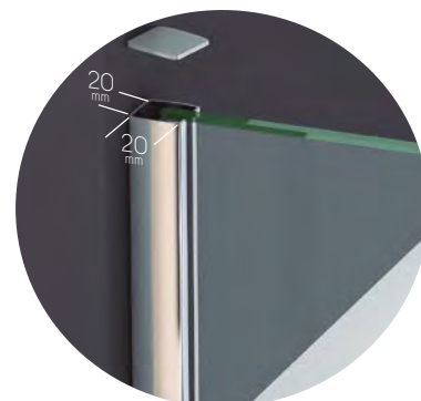
Detalle cerco vertical
