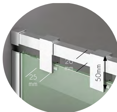
Detalle soporte de barra 180°
