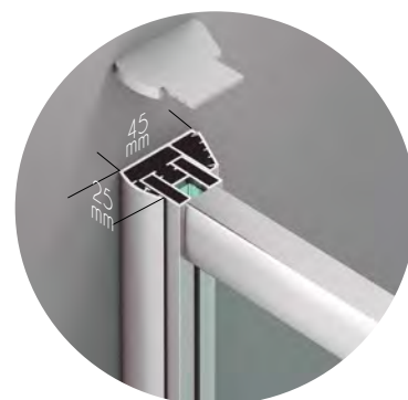
Detalle cerco compensador Riaza Enmarcada
