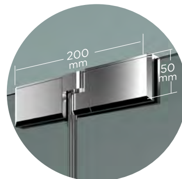
Detalle de bisagra doble
