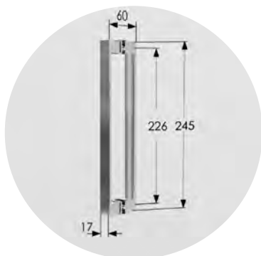
Tirador
