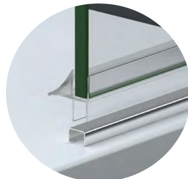
Detalle perfil de estanqueidad
