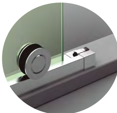
Detalle tope de freno London Sport
