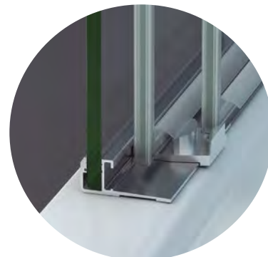
Detalle cerco inferior 2P+F Vista interior
