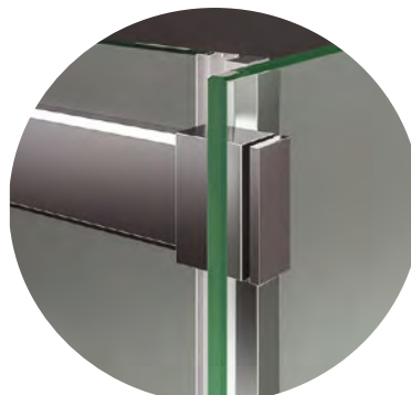
Detalle soporte lateral
