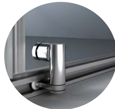
Detalle rodamiento inferior
