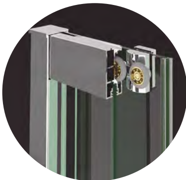
Detalle rodamiento superior
