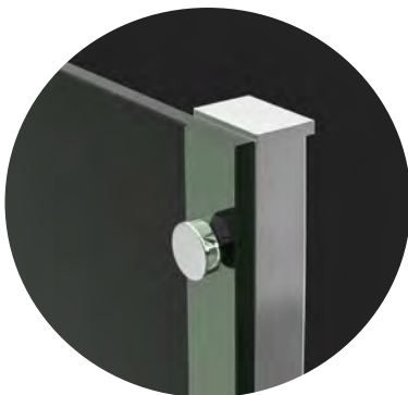
Detalle unión vidrio lateral
